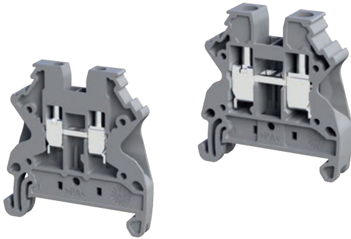
NTB 2,5
